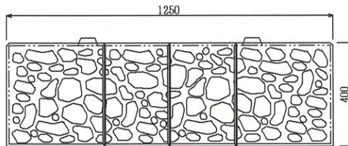
正面図
